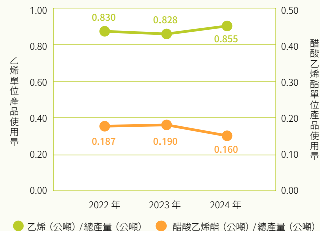
近三年 林園廠單位產品主要原料使用量
